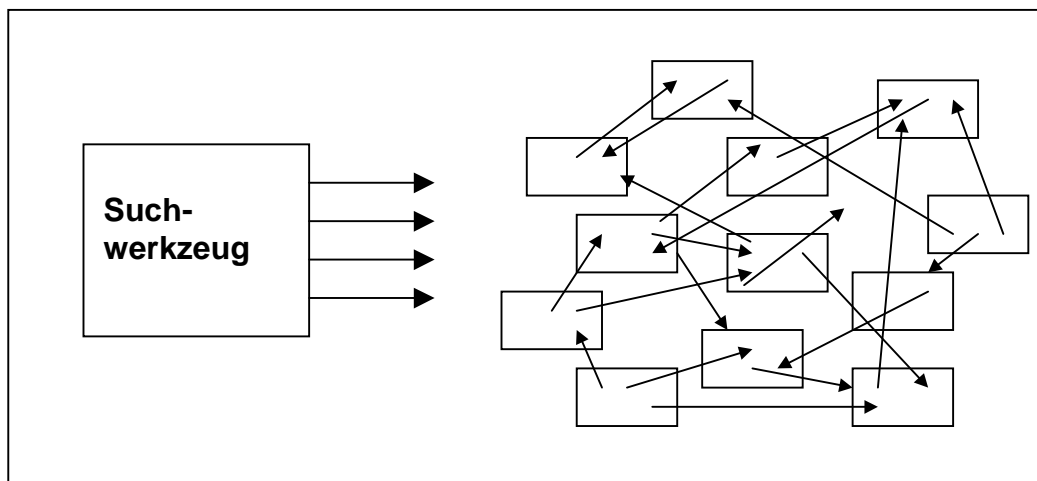
Abbildung 3: Unsequenzierter Hypertext
