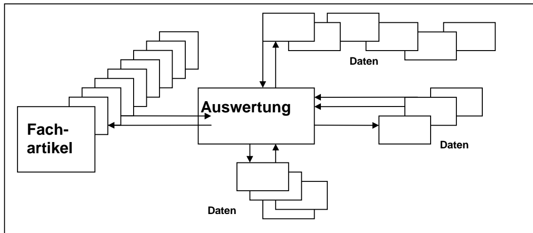
Abbildung 4: monosequenzierter Hypertext
