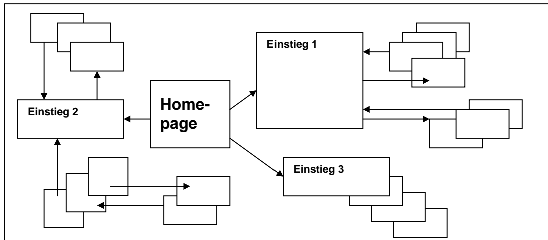
Abbildung 2: Mehrfachsequenzierter Hypertext
