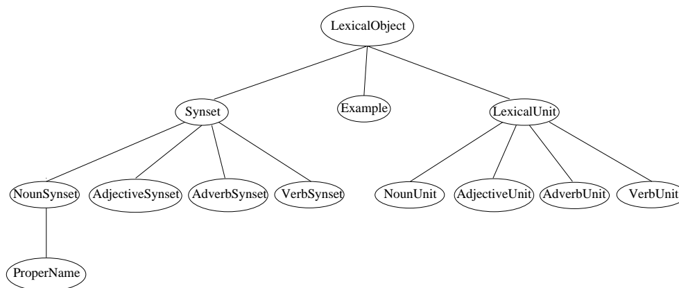
Abbildung 4: Klassenhierarchie für die OWL-Modellierung von GermaNet
