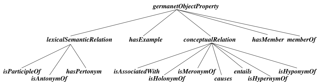
Abbildung 5: Hierarchie der Object Properties für GermaNet
