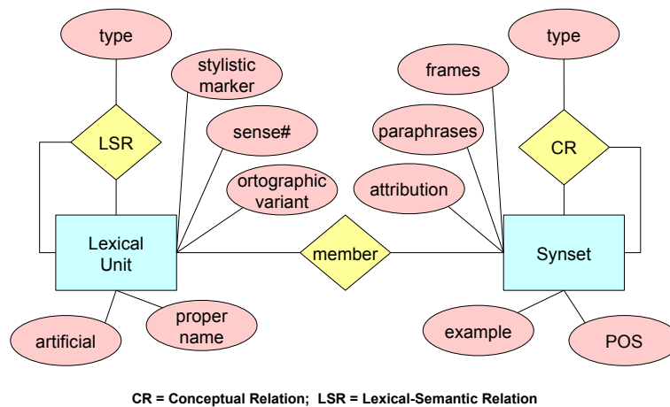
Abbildung 3: Entity-Relationship-Graf GermaNet
